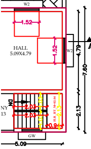
DOOR PLAN
