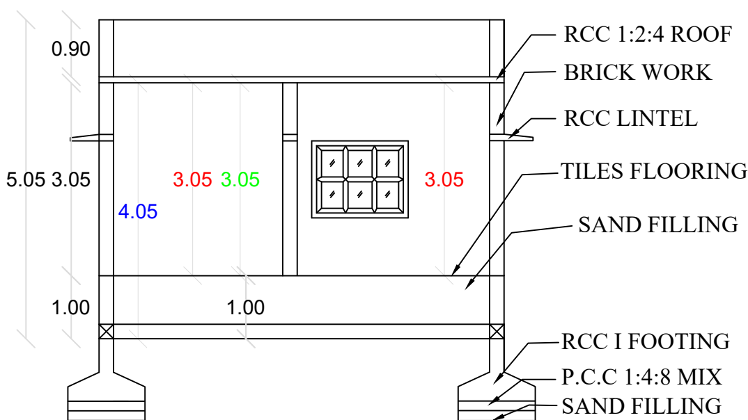
SECTION A-B
