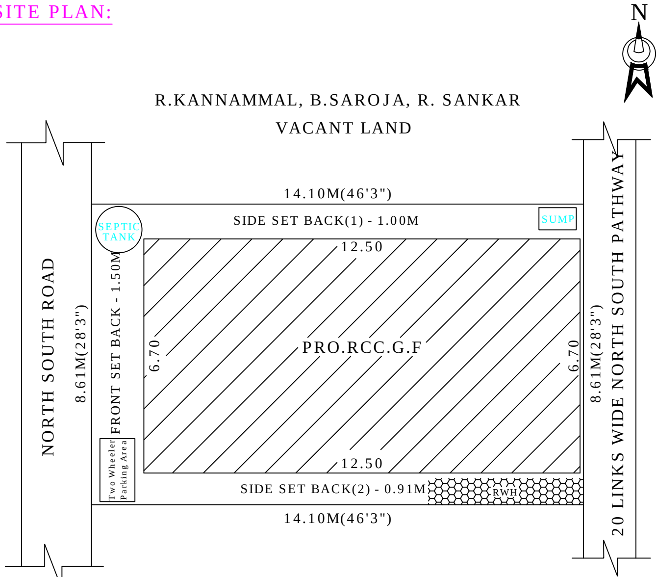
SITE PLAN:
