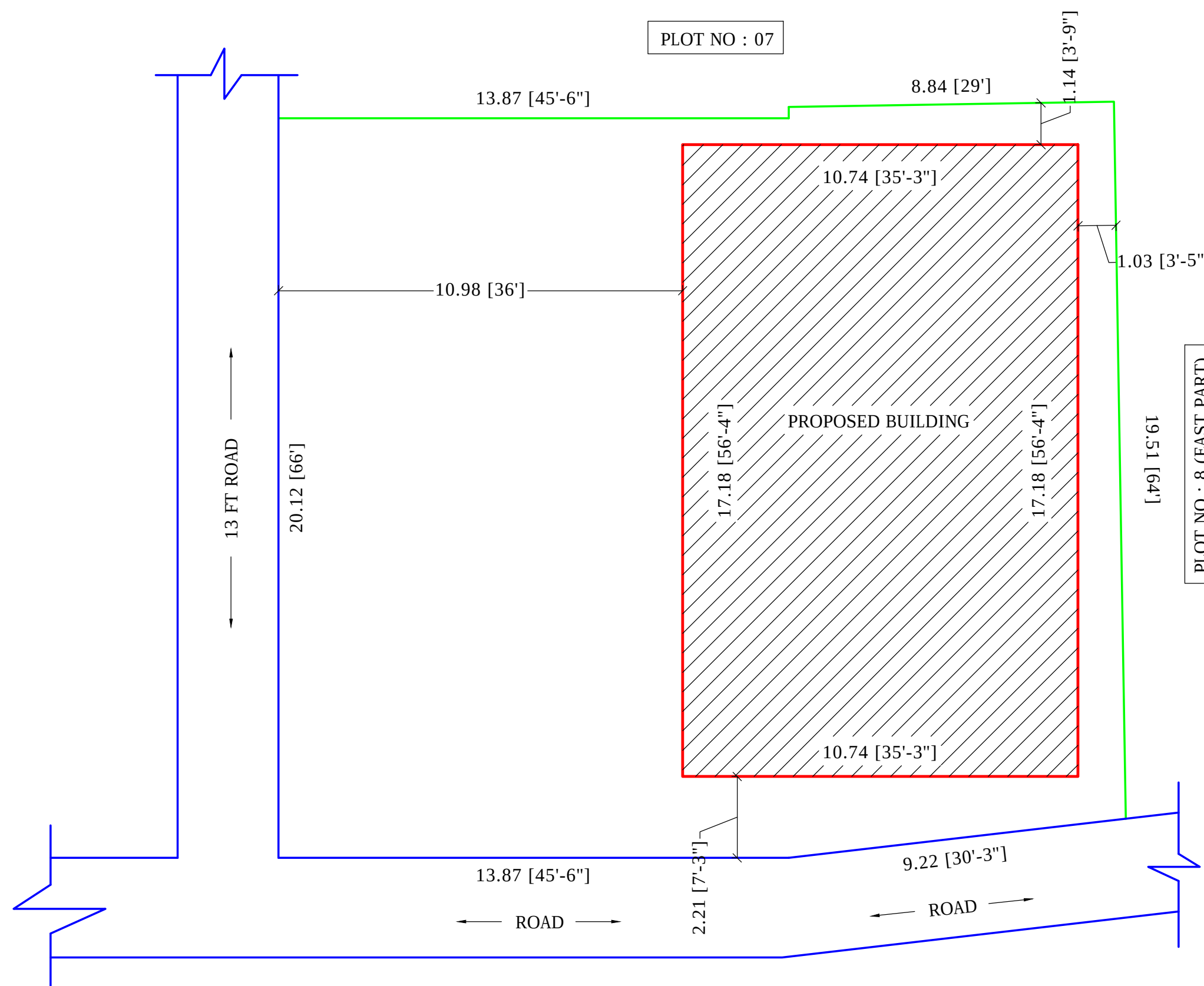
SITE PLAN ( 1: 100)
