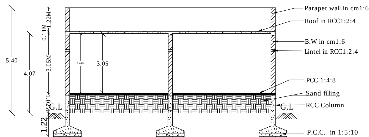
SECTION - AB
