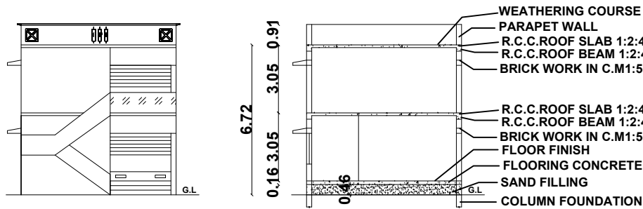
ELEVATION
