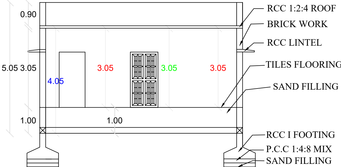
SECTION A-B
