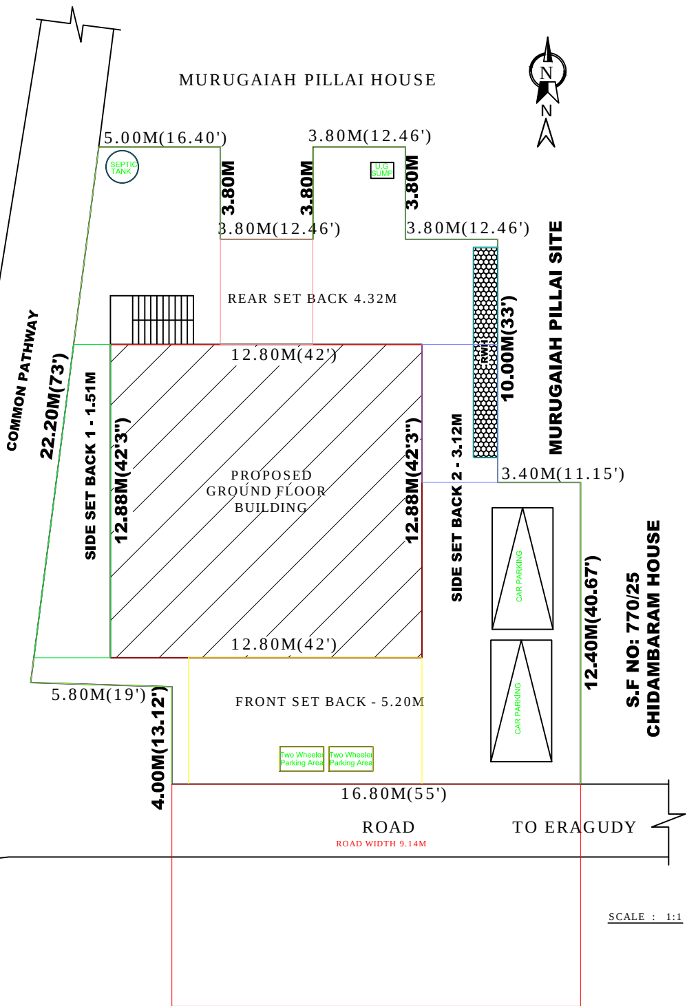
SITE PLAN :
