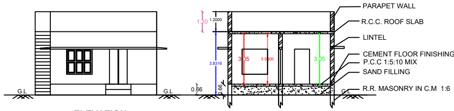
ELEVATION
