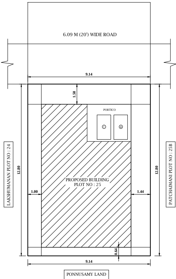
SITE PLAN 1:100
