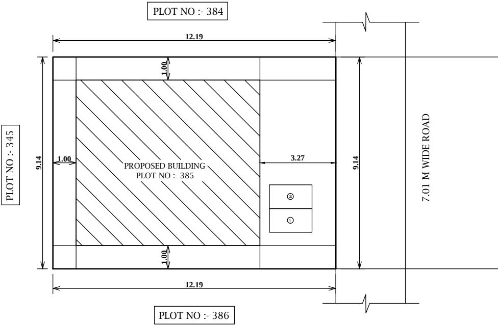
SITE PLAN 1:100
