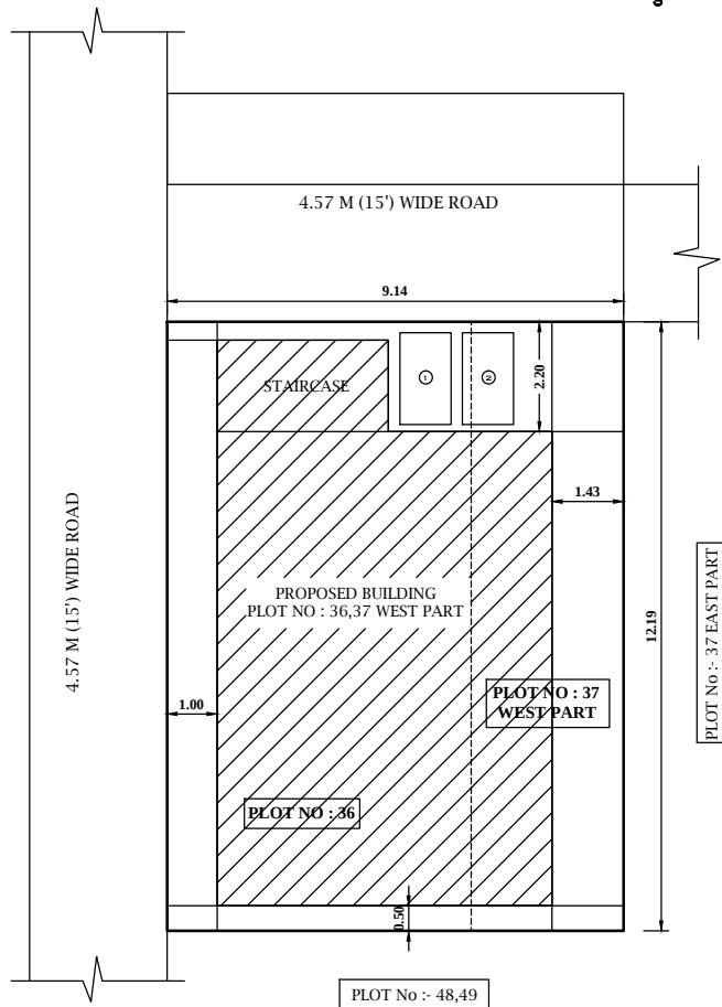
SITE PLAN 1:100
