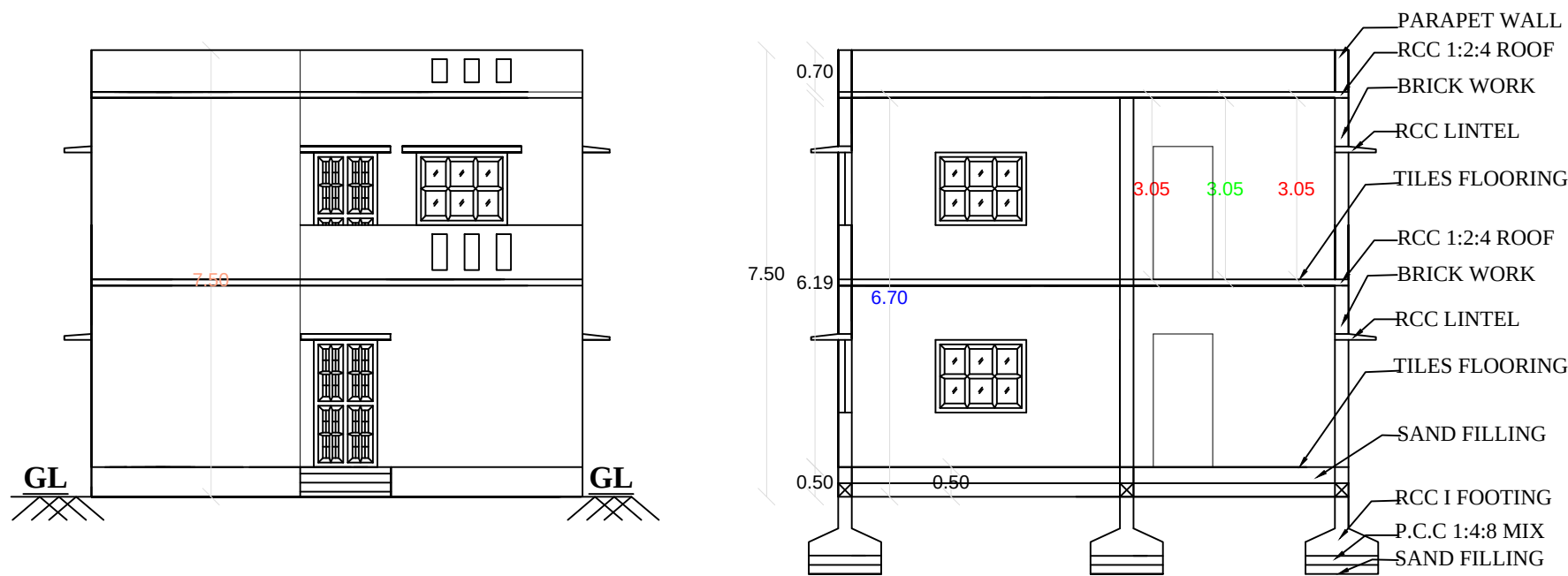
ELEVATION
