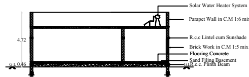
SECTION A-B
