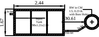
SOAK PIT
