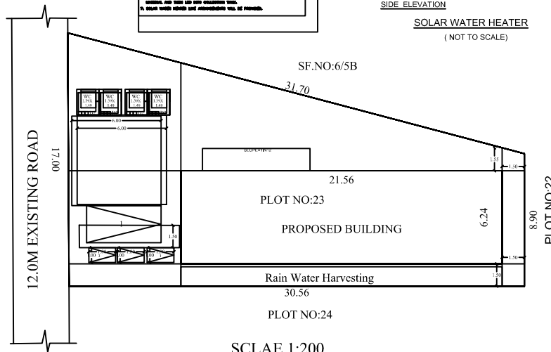
SCLAE 1:200 SITE PLAN
