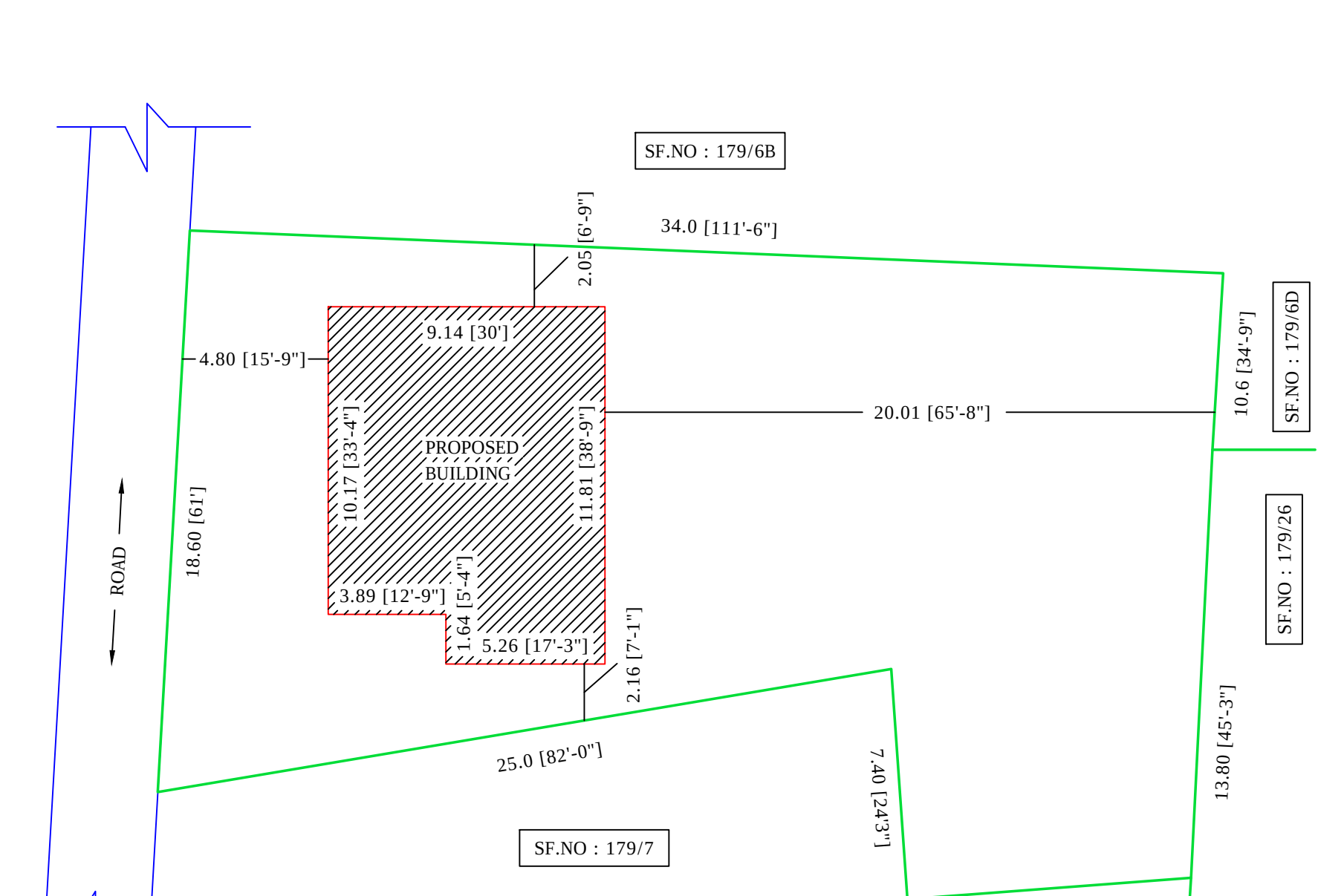
SITE PLAN ( 1:200 )
