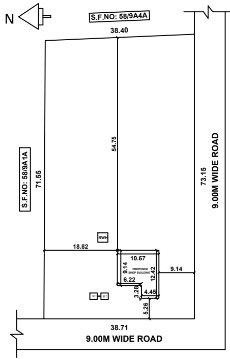
SITE PLAN SCALE: 1:400
