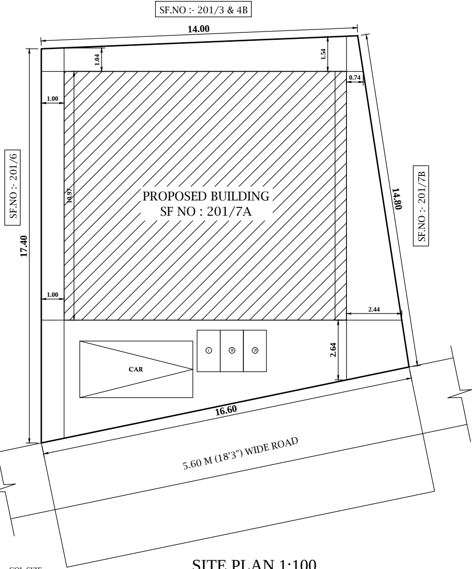
SITE PLAN 1:100
