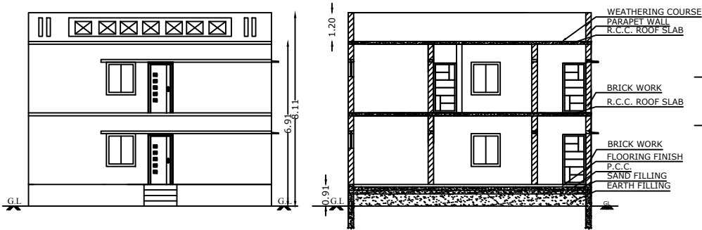
ELEVATION
