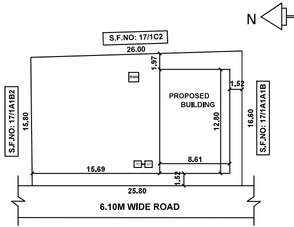
SITE PLAN SCALE: 1:400
