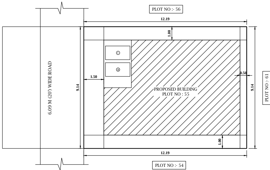
SITE PLAN 1:100
