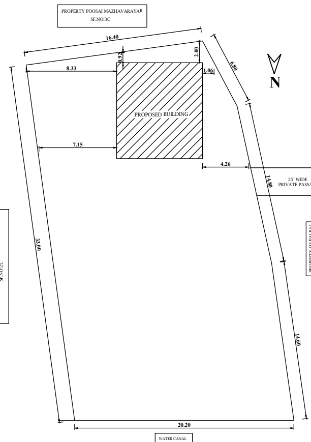
SITE PLAN (SCALE-1:150)
