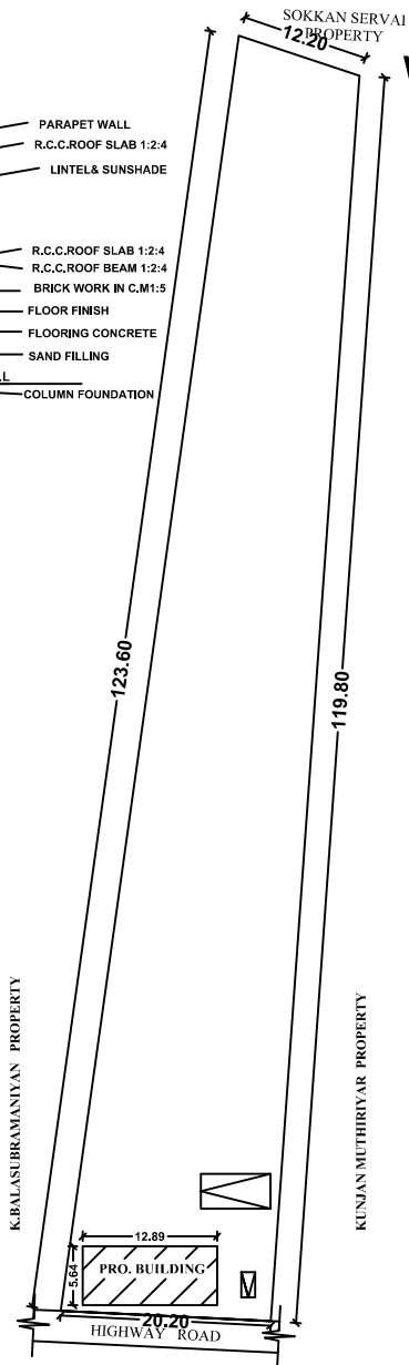
SITE PLAN ( SCALE 1: 100)
