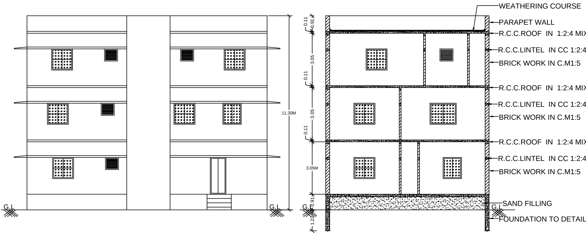
ELEVATION
