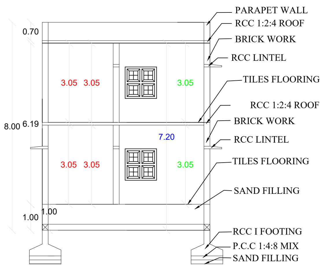
SECTION A-B
