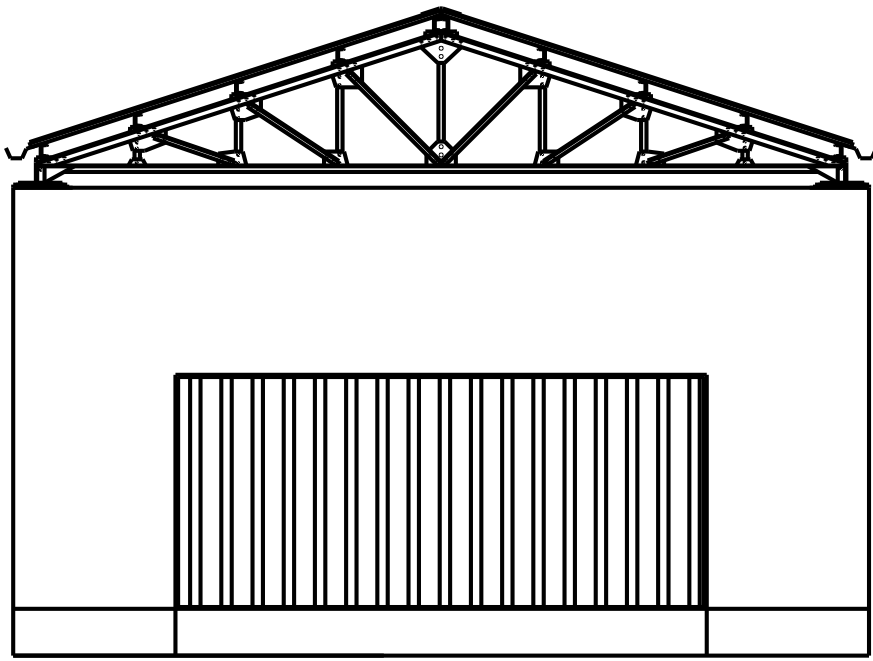
ELEVATION - A
