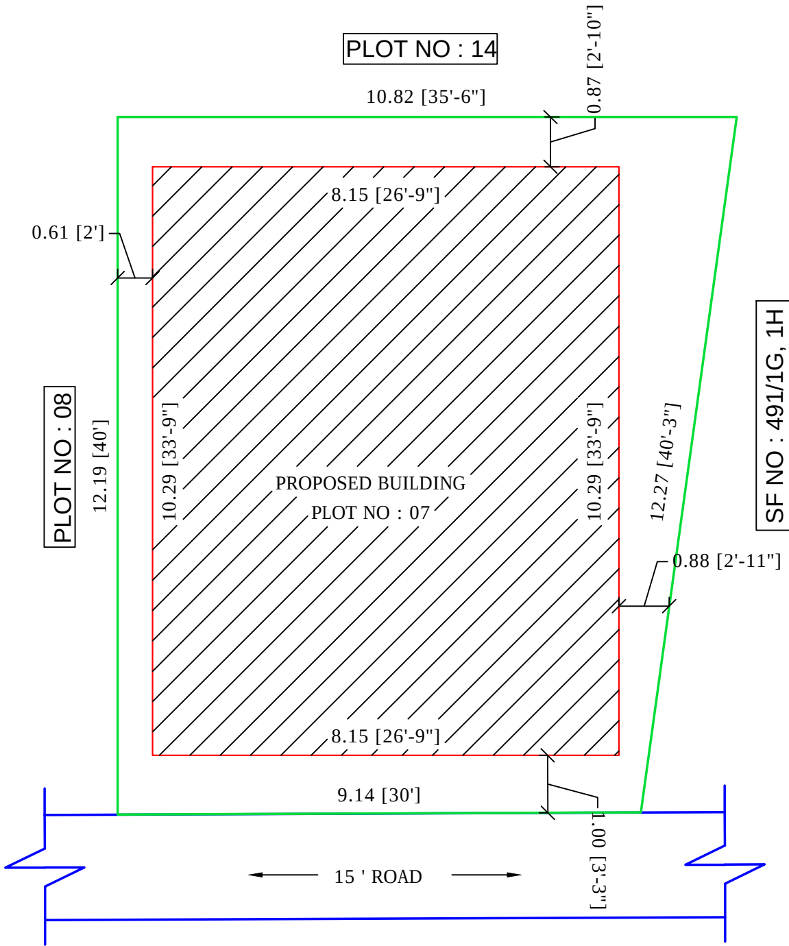
SITE PLAN ( 1:100 )
