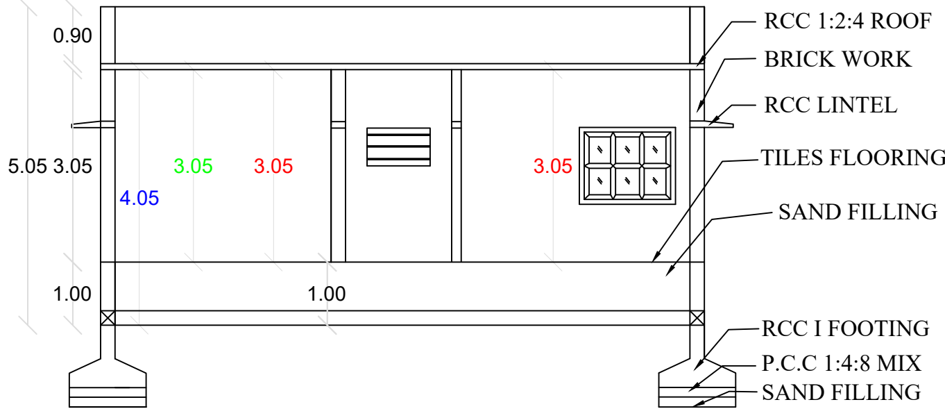
SECTION A-B
