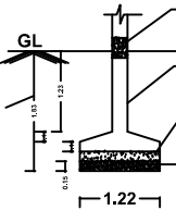
FOUNDATION DE
