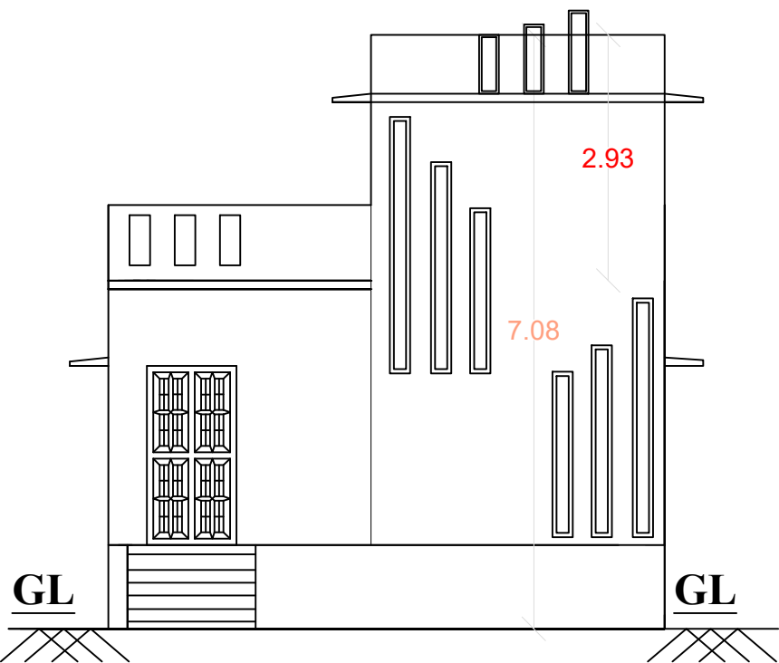
ELEVATION
