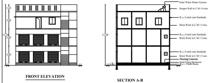
SECTION A-B
