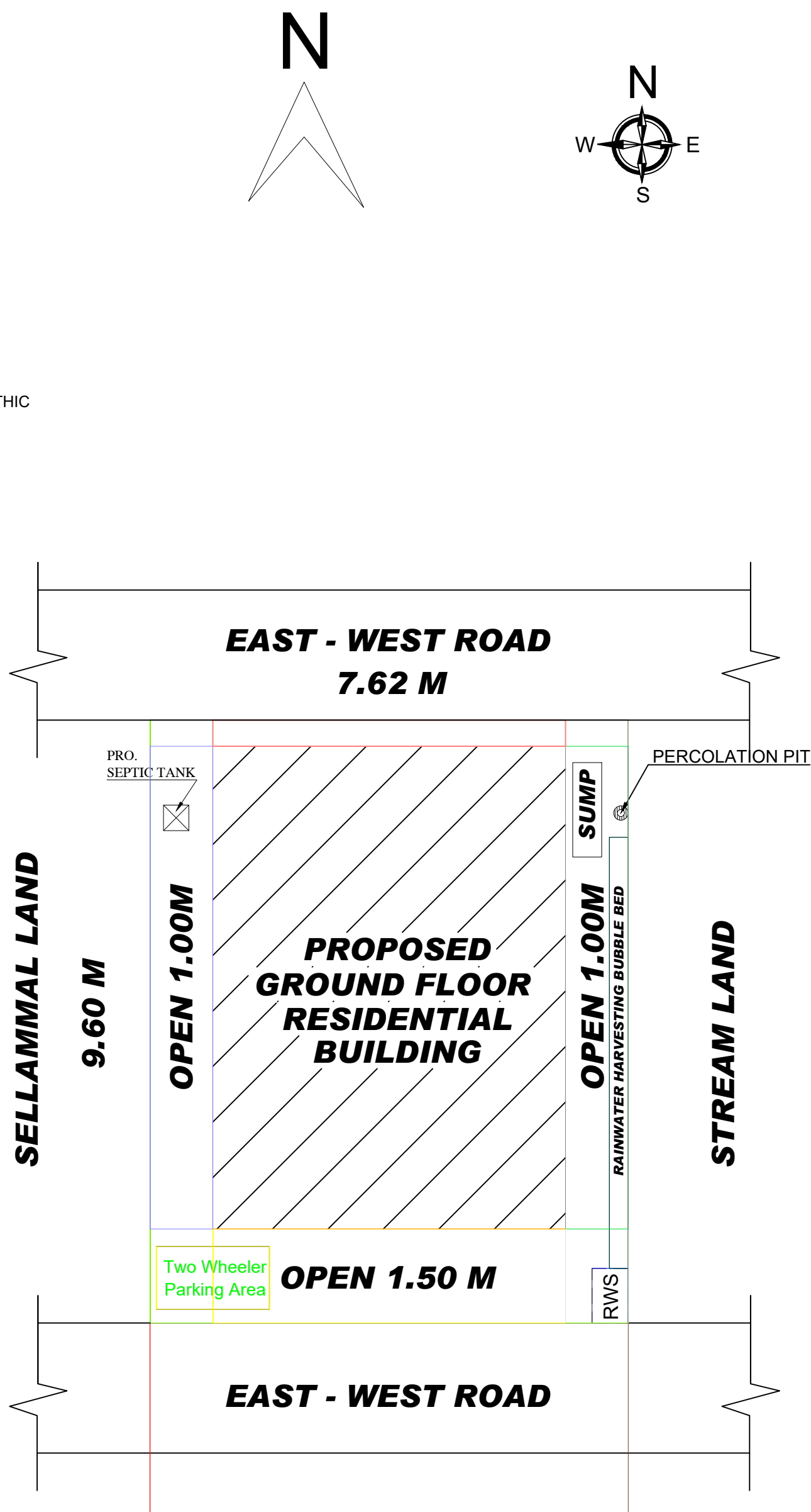
SITE PLAN (SCALE: 1:1)
