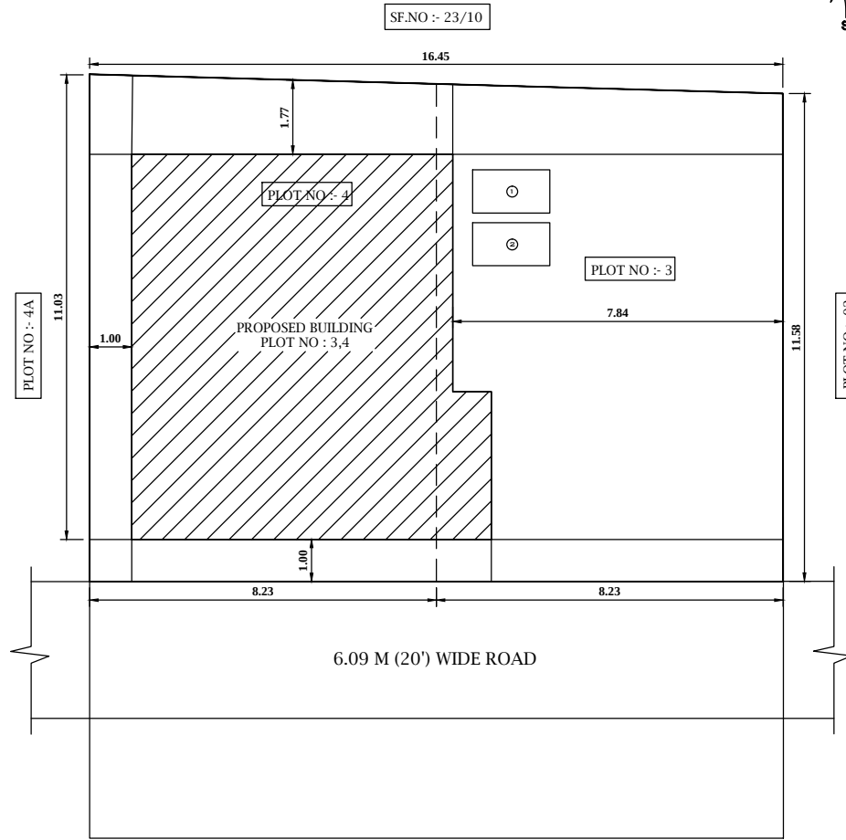
SITE PLAN 1:100
