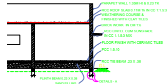
ON 'A - A'
