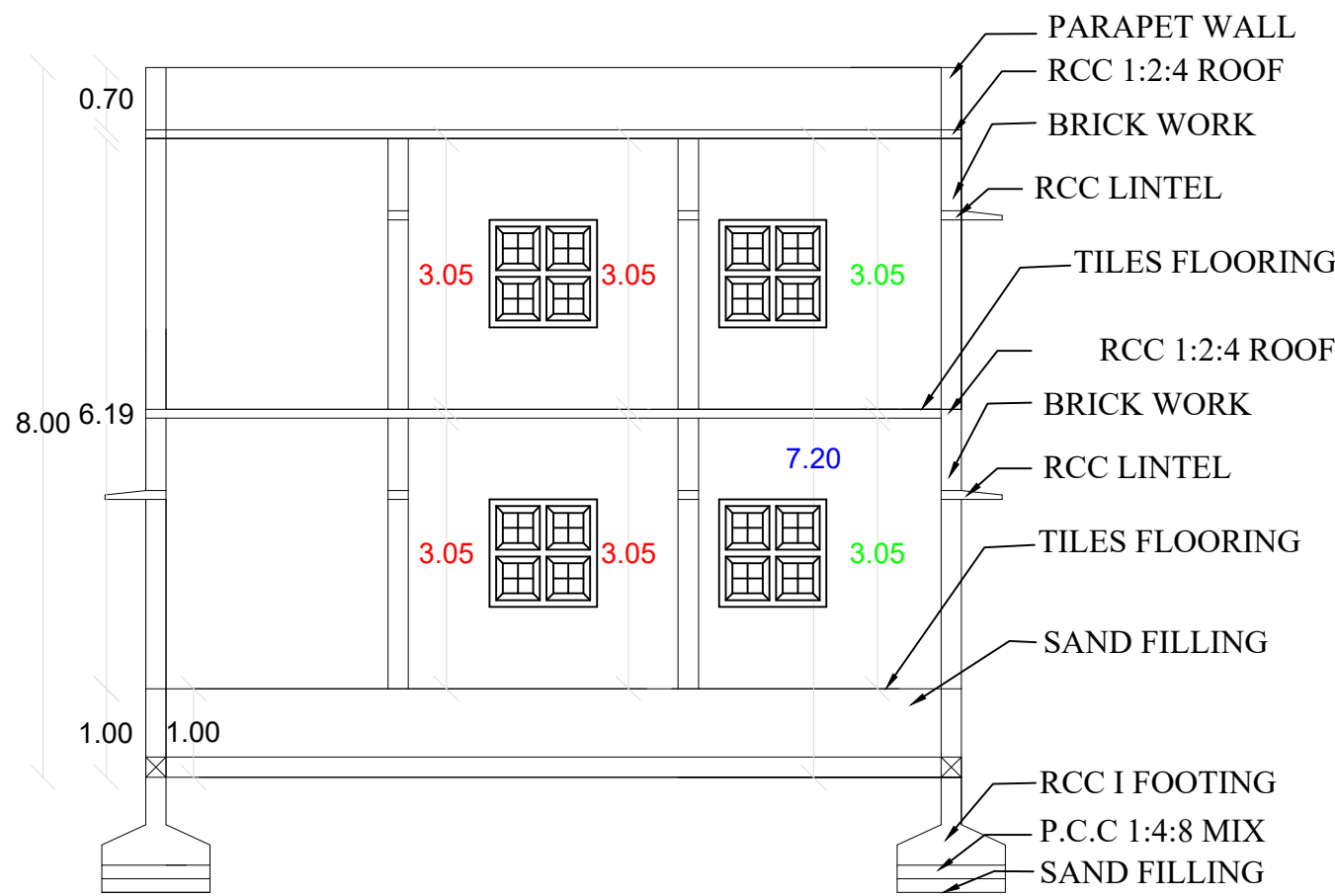
SECTION A-B
