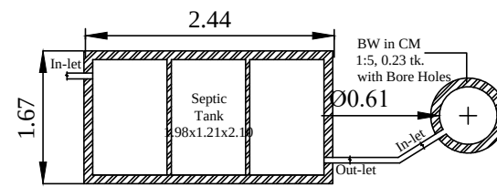
SOAK PIT
