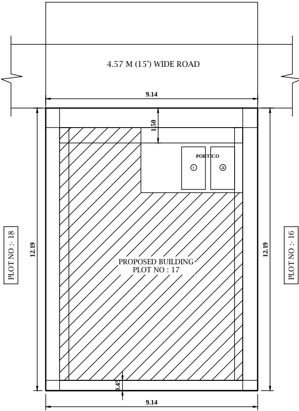
SITE PLAN 1:100
