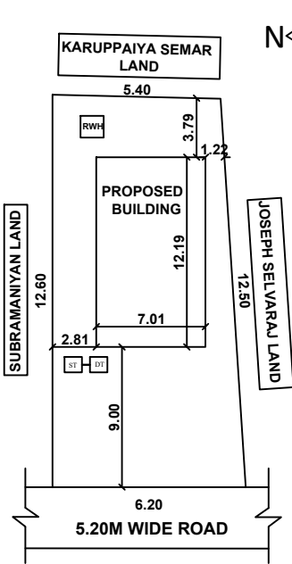
SITE PLAN SCALE: 1:200
