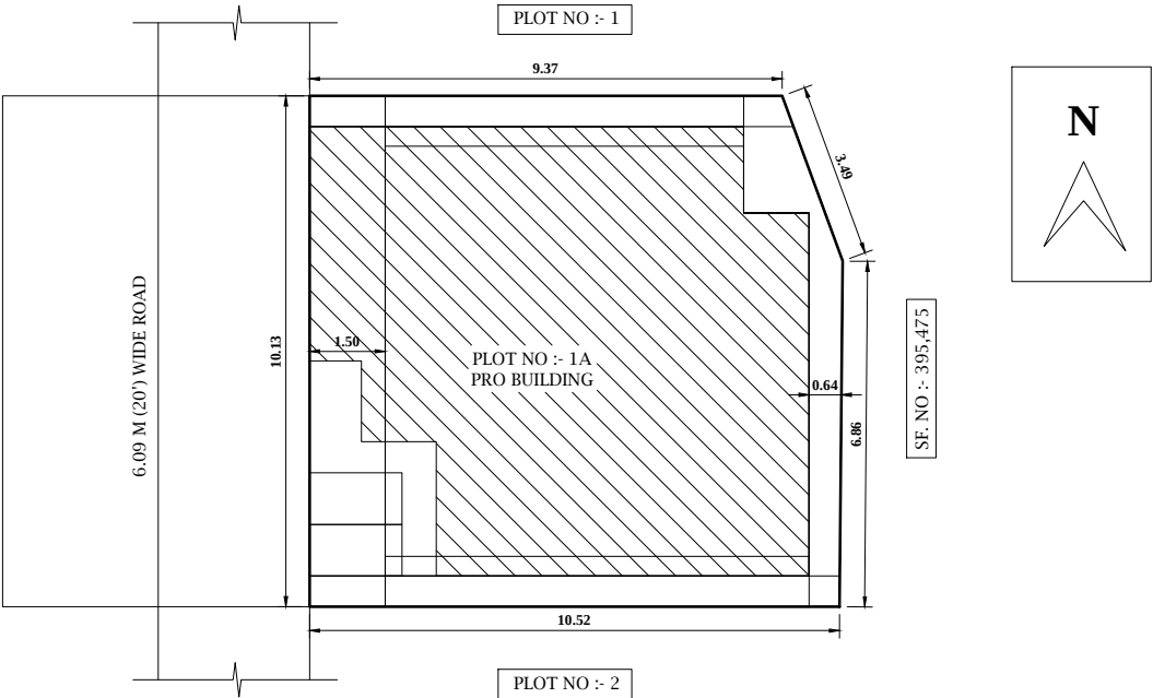
SITE PLAN 1:100
