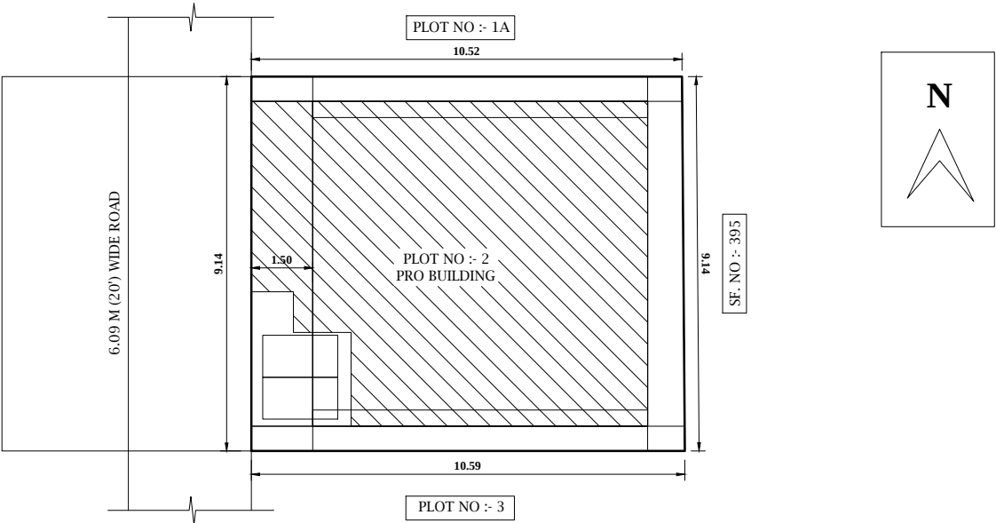
SITE PLAN 1:100
