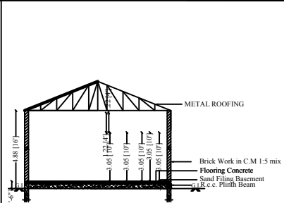
SECTION A-B
