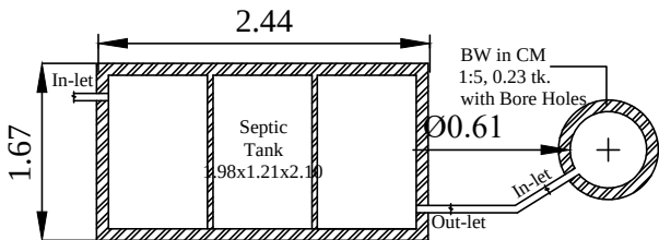
SOAK PIT
