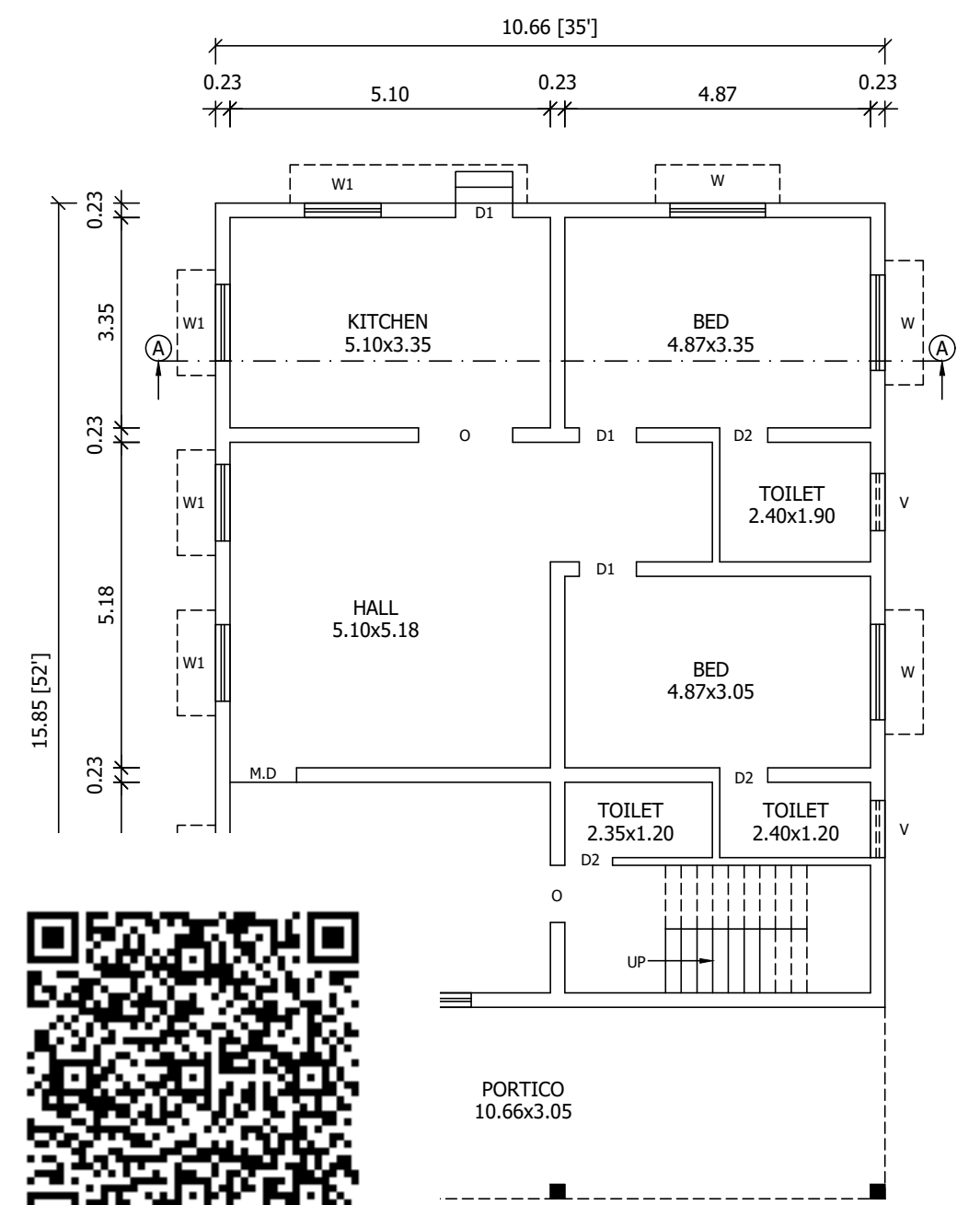
UND FLOOR PLAN
