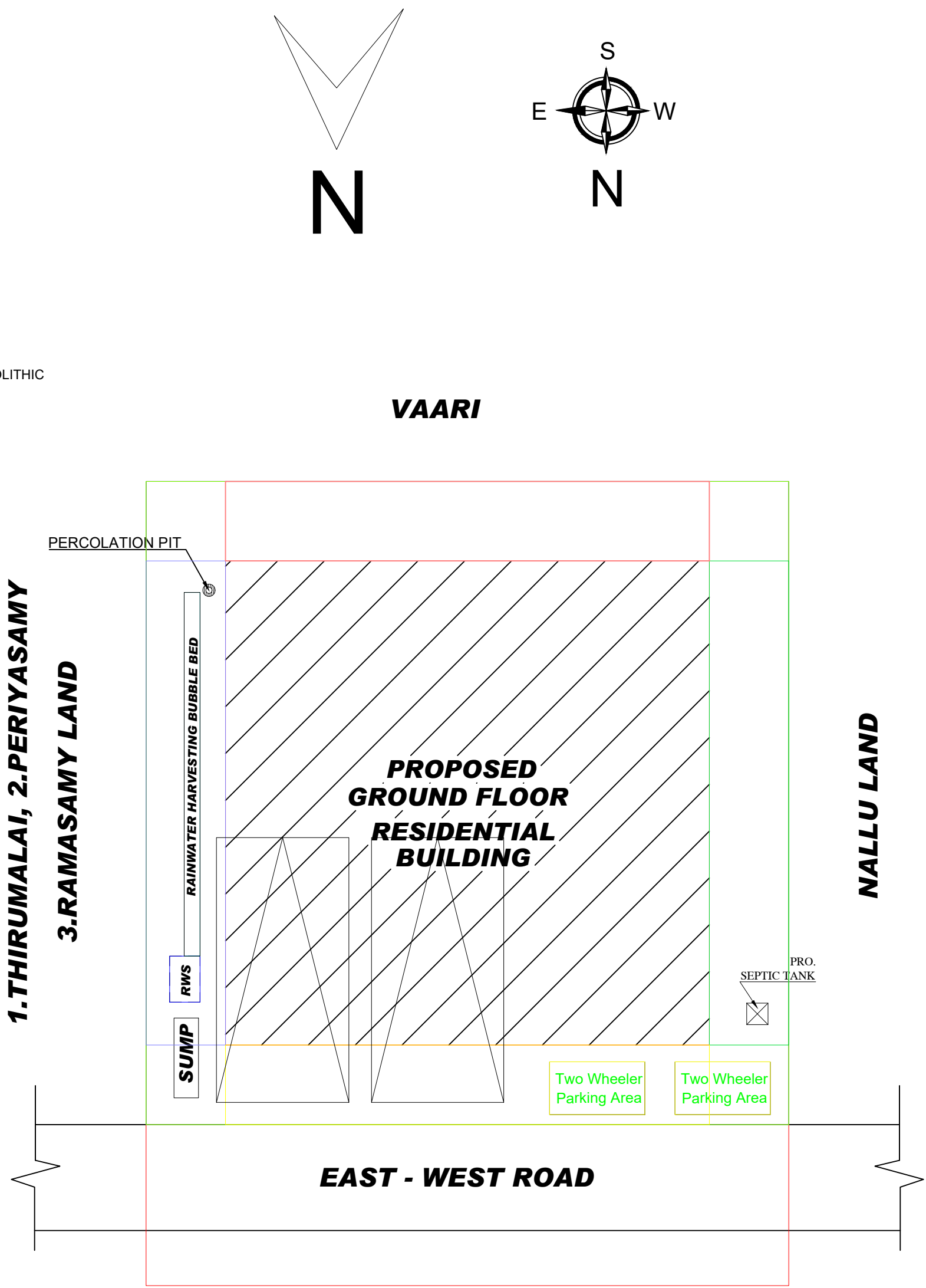
SITE PLAN (SCALE: 1:1)
