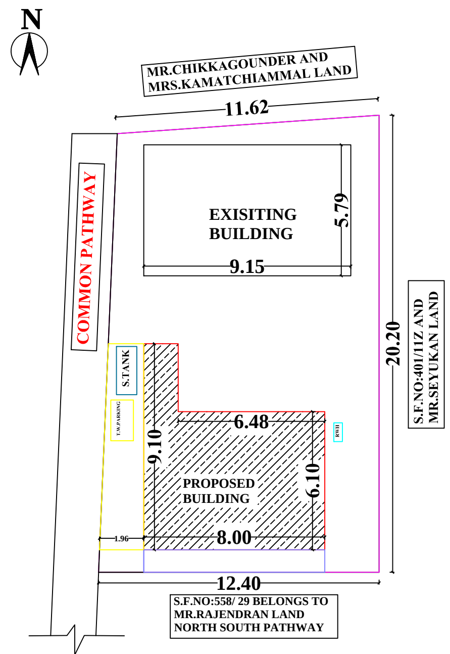
SITE PLAN:-
