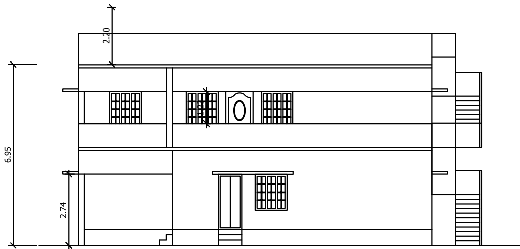
ELEVATION
