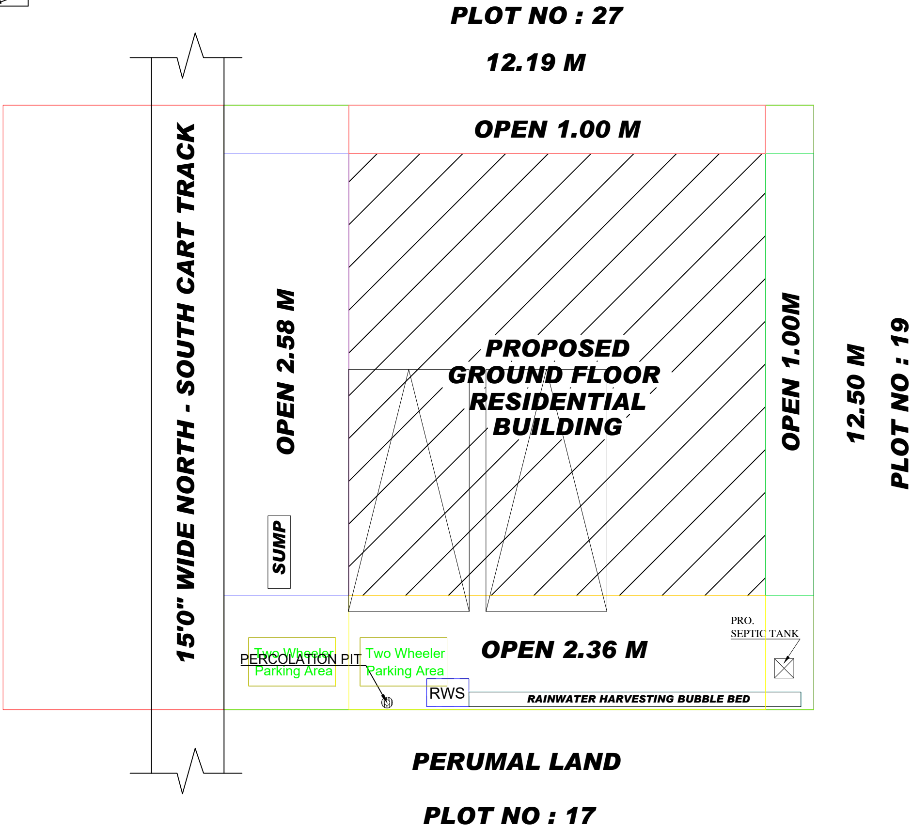
SITE PLAN (SCALE: 1:1)
