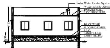
SECTION A-B
