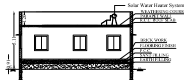
SECTION A-B
