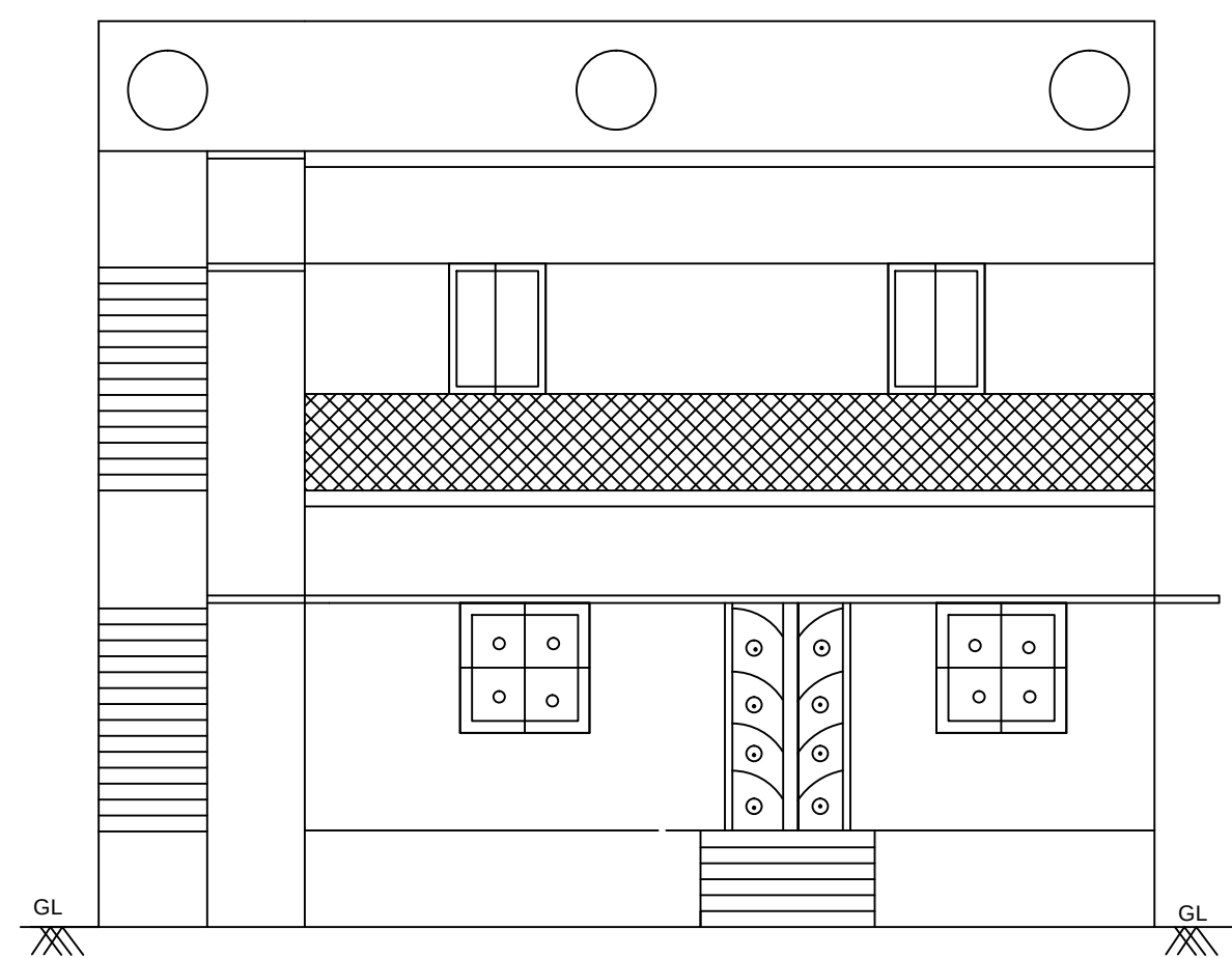
ELEVATION
